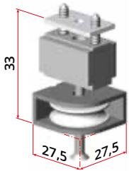
art. 2735 per/for art. 2201 - 5801 Puleggia terminale da fissare al binario End pulley with hooking for the rail
