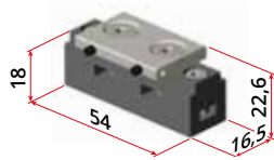
art. 2742 per/for art. 2441 Inserto di fissaggio con fermacavo 2758 su 2441 Fixing insert with cable-stop 2758 on 2441
