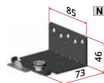
Art. 2006/30/DX/N Guida inferiore destra per anta esterna spessore 30 mm Right lower guide for external door thickness 30 mm
