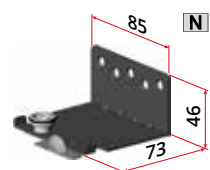
Art. 2006/30/SX/N Guida inferiore sinistra per anta esterna spessore 30 mm Left lower guide for external door thickness 30 mm
