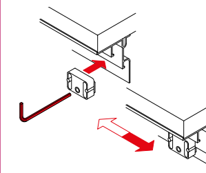
Art. 2008 Fermo inferiore da fissare al binario, inseribile e regolabile frontalmente.
