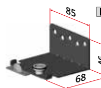
Art. 2006/25/DX/N Guida inferiore destra per anta esterna spessore 25 mm Right lower guide for external door thickness 25 mm
