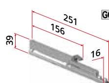
art. 5357/S Fermo superiore ammortizzato, corsa 55 mm, funzionamento ad olio silconico, versione premium Upper soft close, 55 mm stroke, operating with silicone oil, premium version
