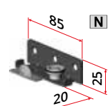
Art. 2004/DX/N Guida inferiore destra per anta interna Right lower guide for internal door
