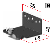
Art. 2006/25/SX/N Guida inferiore sinistra per anta esterna spessore 25 mm Left lower guide for external door thickness 25 mm
