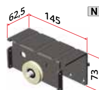
Art. 1905/25/N Carrello superiore ambidestro per anta esterna spessore 25 mm Upper carriage for external door thickness 25 mm
