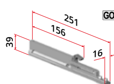
art. 5357 Fermo superiore ammortizzato, corsa 55 mm, funzionamento ad olio silconico Upper soft close, 55 mm stroke, operating with silicone oil
