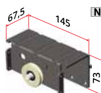
Art. 1905/30/N Carrello superiore ambidestro per anta esterna spessore 30 mm Upper carriage for external door thickness 30 mm
