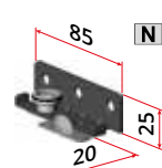
Art. 2004/SX/N Guida inferiore sinistra per anta interna Left lower guide for internal door
