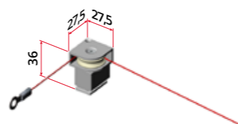
Art. 5151 per/for art. 5301 Ruota di rinvio da fissare al binario 5301 adatto alle ante interne ed esterne, per Serie 5300 Return wheel to be fixed to the rail art. 5301 and suitable for internal and external doors. For serie 5300
