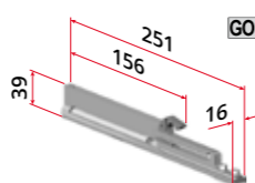
Art. 5357 Fermo superiore SX / DX ammortizzato, corsa 55 mm, funzionamento ad olio silconico. Per serie 2000 e 5300 Upper stop shock-absorbed L / R, 55 mm stroke. Working with silicone oil. For series 2000 and 5300
