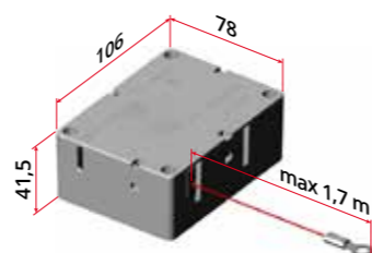
Art. 5101/80 Meccanismo di richiusura a molla con ammortizzatore per ante fino a 80 Kg Corsa massima 170 cm Reclosing spring system with shock-absorber suitable for door with capacity up to 80 Kg. Maximum stroke 170 cm
