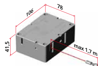
Art. 5101/60 Meccanismo di richiusura a molla con ammortizzatore per ante fino a 60 Kg Corsa massima 170 cm Reclosing spring system with shock-absorber suitable for door with capacity up to 60 Kg. Maximum stroke 170 cm
