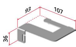
Art. 5106/SX per/for art. 2003/SX Staffa di aggancio del cavo di trascinamento per il carrello dell'anta interna sinistra per serie 2000 Carriage dragging cable hooking bracket of the left internal door for serie 2000
