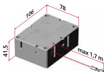
Art. 5101/40 Meccanismo di richiusura a molla con ammortizzatore per ante fino a 40 Kg Corsa massima 170 cm Reclosing spring system with shock-absorber suitable for door with capacity up to 40 Kg. Maximum stroke 170 cm
