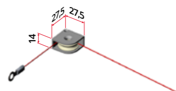
Art. 5115 Ruota di rinvio per applicazioni universali dell'art. 5101 Return wheel for universal applications of art. 5101
