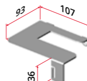
Art. 5106/DX per/for art. 2003/SX Staffa di aggancio del cavo di trascinamento per il carrello dell'anta interna destra per serie 2000 Carriage dragging cable hooking bracket of the right internal door for serie 2000
