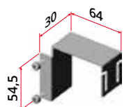
Art. 5103 per/for art. 2005/SX - 2005/DX Staffa di aggancio del cavo di trascinamento per il carrello dell'anta esterna per serie 2000 Carriage dragging cable hooking bracket of the external door for serie 2000
