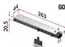
Art. 5373 per/for art. 5303 - 5305 Fermo superiore ammortizzato ad aria, corsa 70 mm. Per serie 5300 Upper stop shock-absorbed, 70 mm stroke, working with air For series 5300
