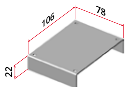
Art. 5109 per/for art. 5001 Staffa di supporto per il fissaggio dell'art. 5101 sulla parte superiore del mobile, per serie 2000 Support bracket for fixing art. 5101 on the furniture top, for serie 2000
